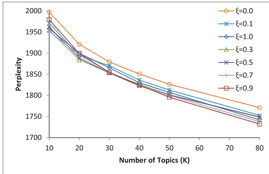
(b) Parameter Study on Twitter for RankTopic
