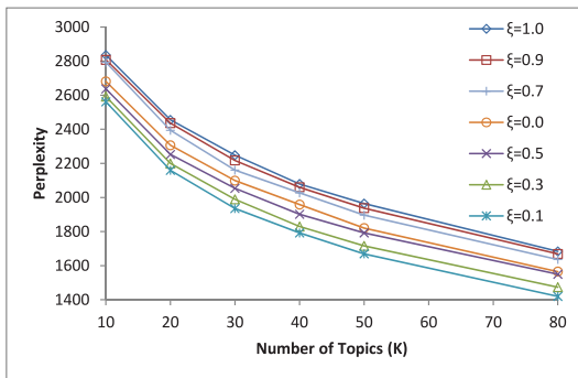
(a) Parameter Study on ArnetMiner for RankTopic
